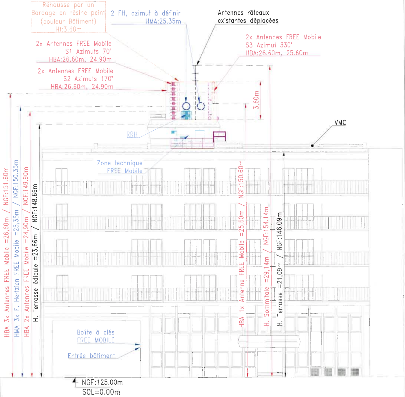
Elévation Façade NORD EST
